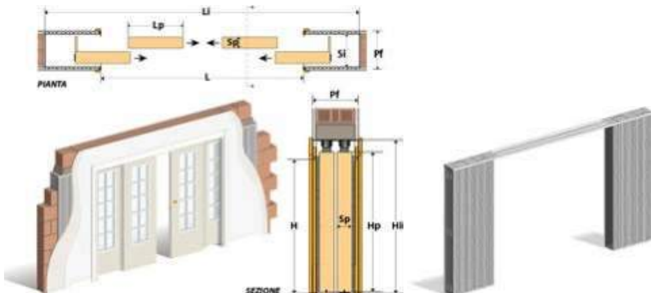
כיס כפול לפתח כפול - ארבע דלתות
