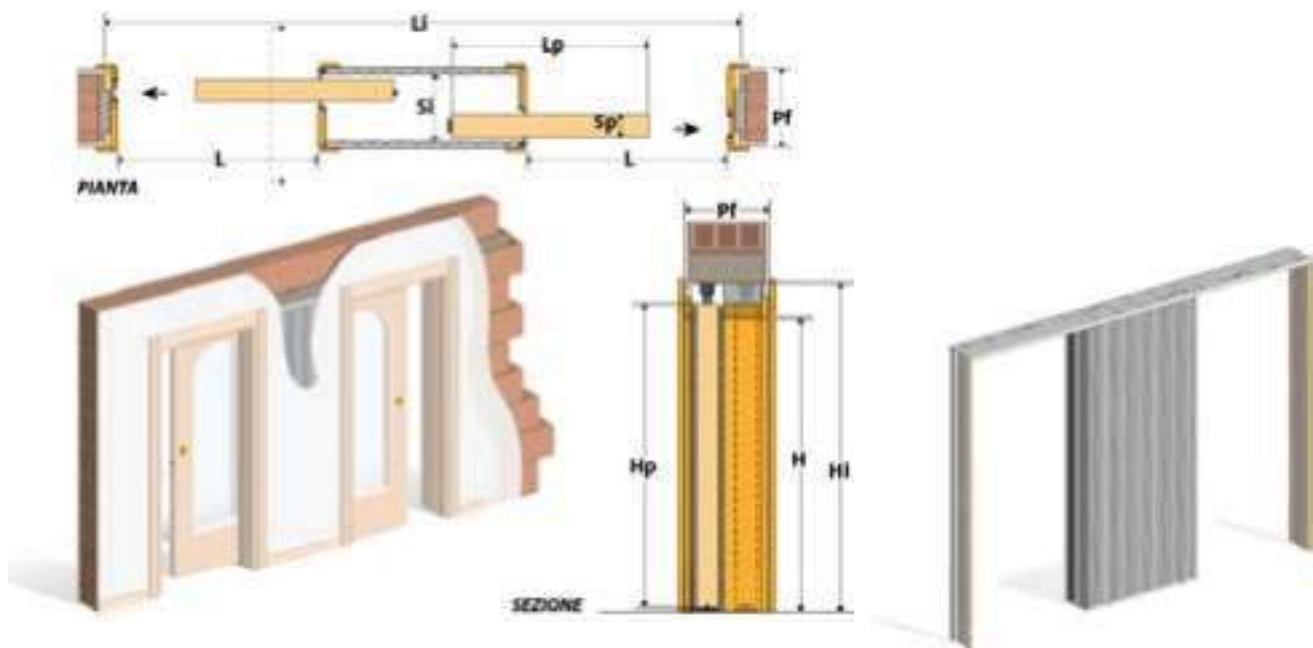
פרט לכיס בודד עם 2 דלתות נגרות נפתחות לצדדים מנוגדים
