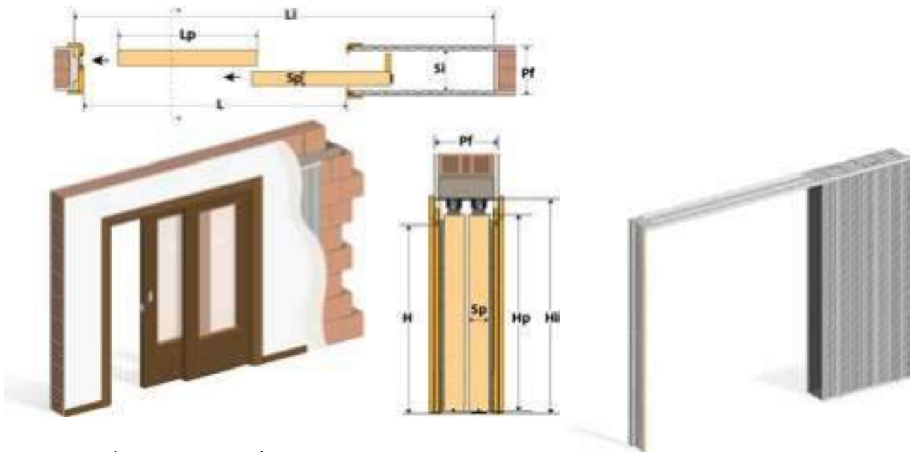
כיס בודד עם שתי דלתות נגררות
