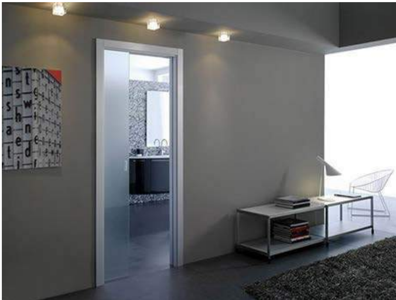
דלתות הזזה לכיס - כנף זכוכית
